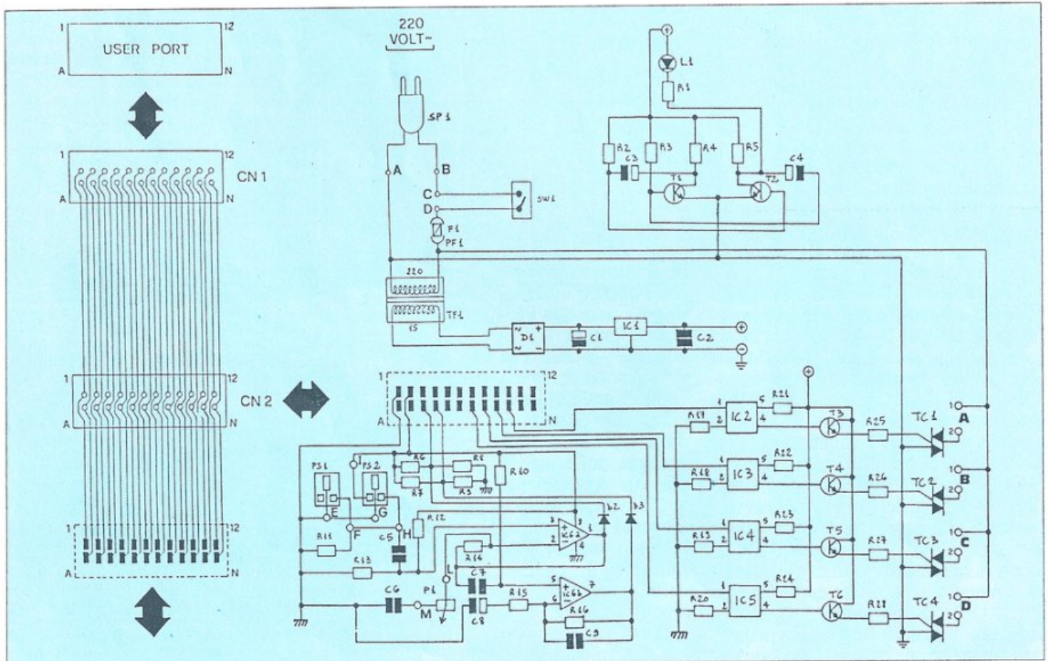
Figura 1. Schema circuitale.
